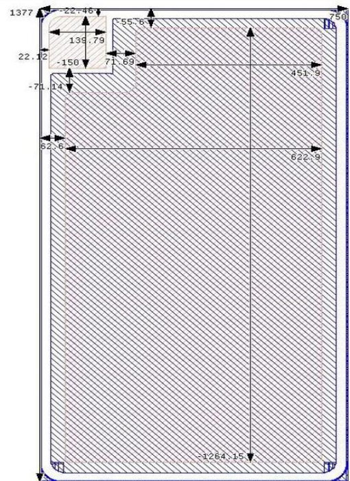
diesize: 810 X 1437
